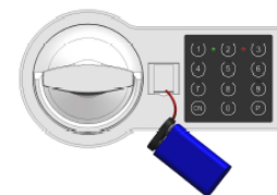
рис. 3. Подключение внешней батареи
